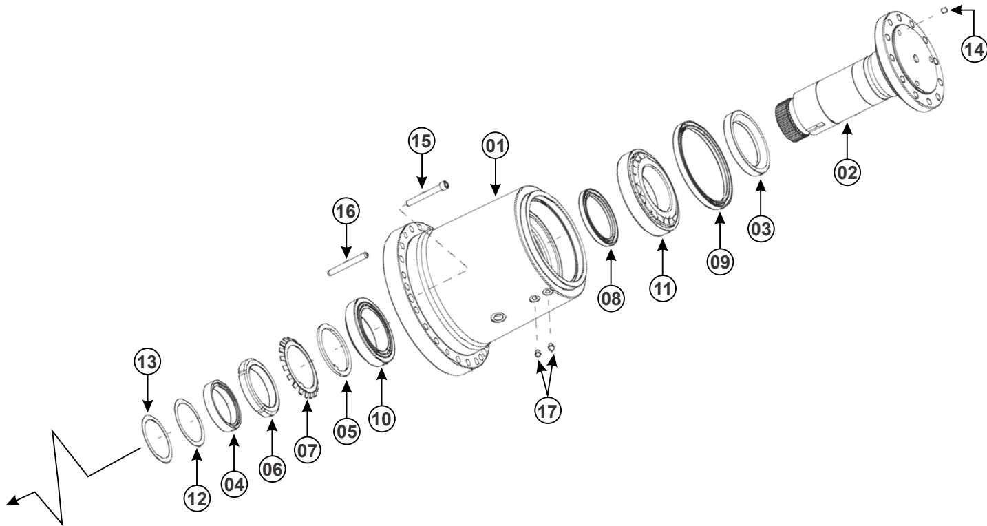
FIGURA 1 - Caixa de Transmissão Brevini ESC 1102 DCS Cód:99.01.0750
